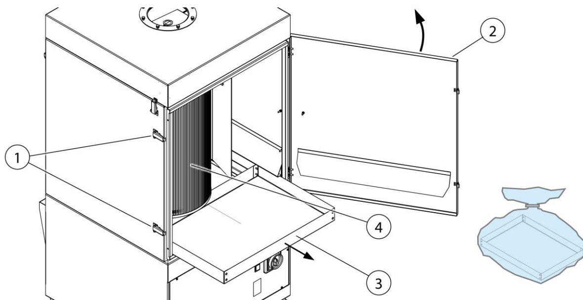
Fig. 7: Svuotamento del collettore di polvere
