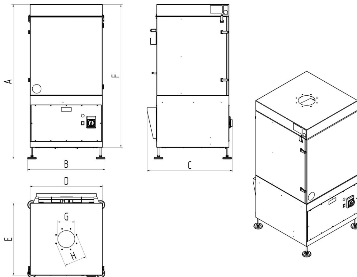
Fig. 13: Disegno quotato
