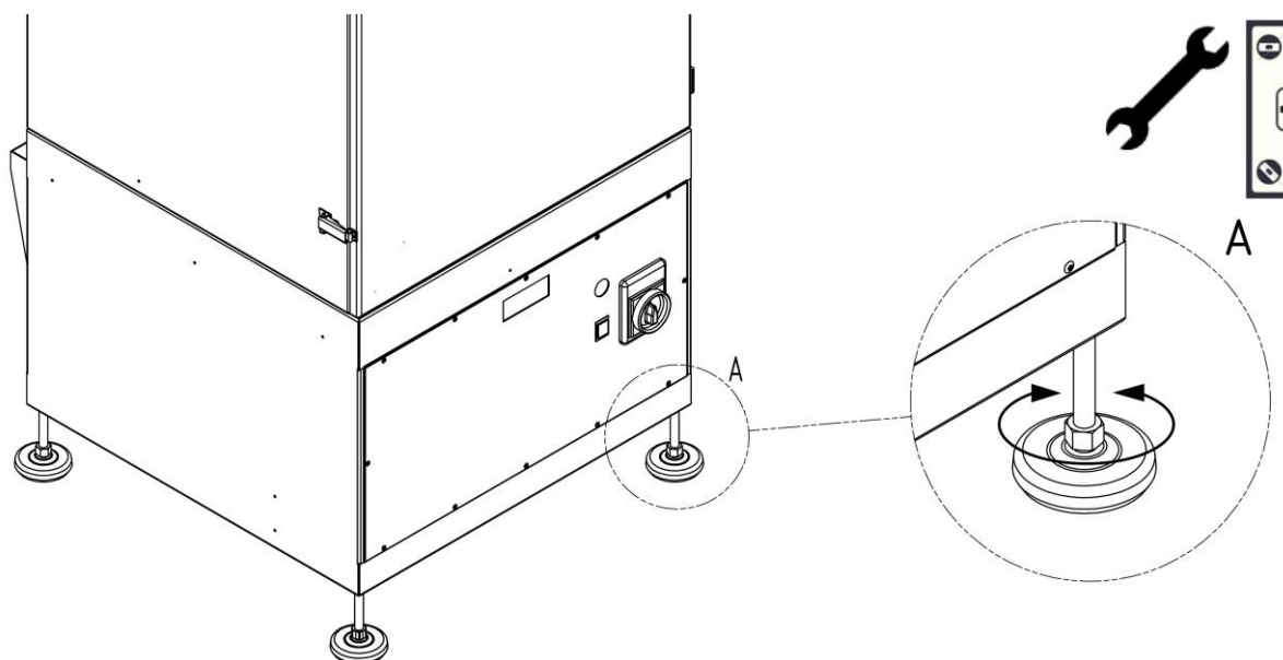
Fig. 2: allineamento del prodotto
