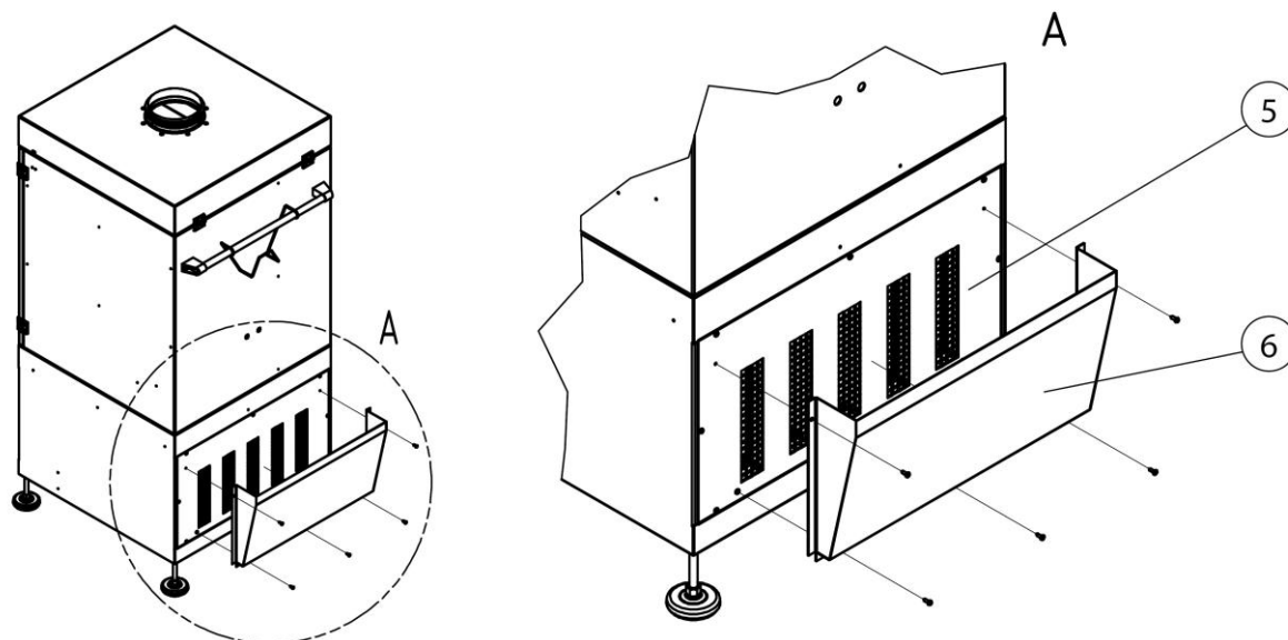
Fig. 4: Montaggio alloggiamento di scarico
