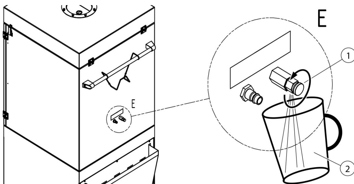
Fig. 8: Scaricare la condensa
